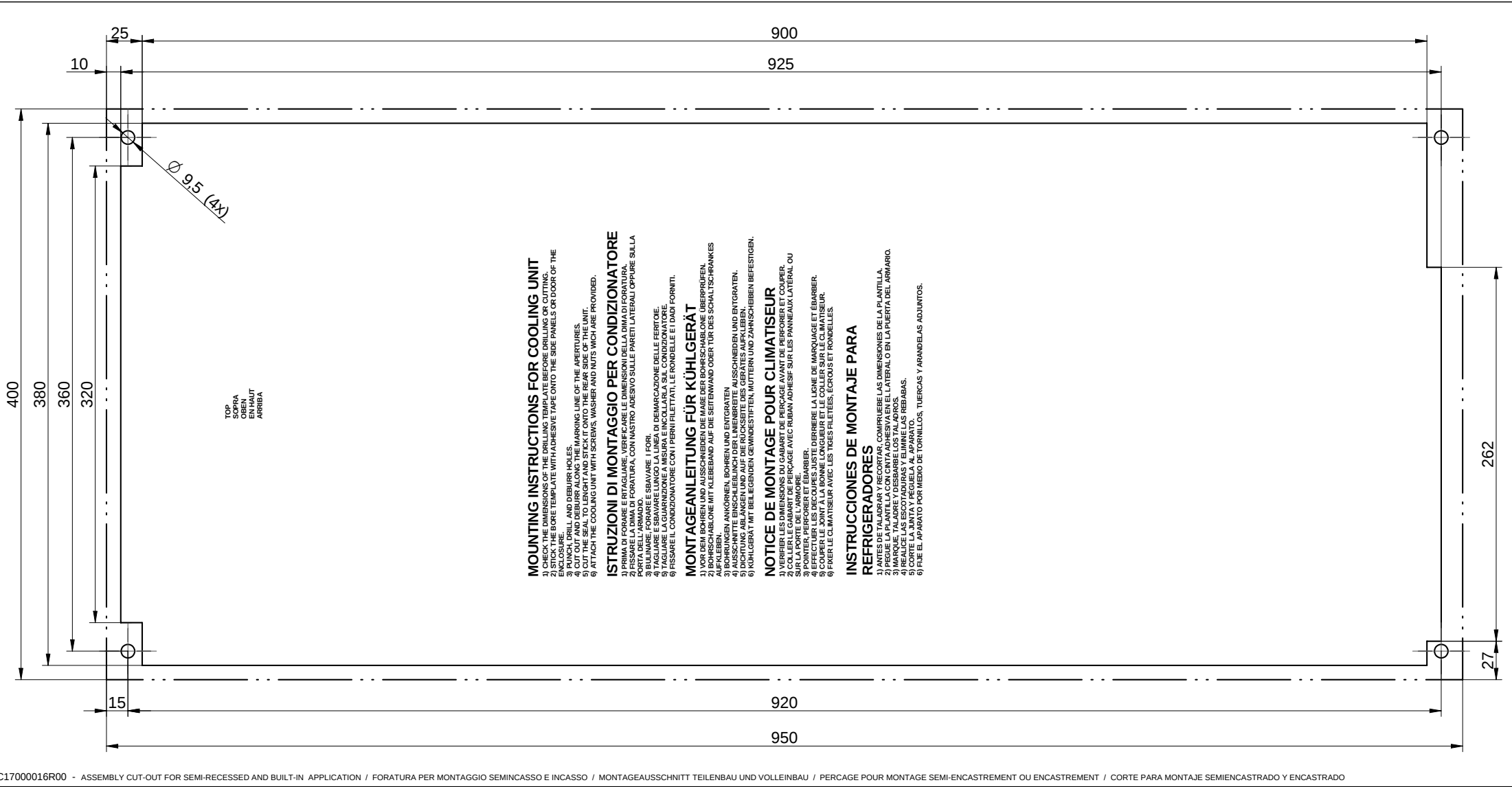
C17000016R00 - ASSEMBLY CUT-OUT FOR SEMI-RECESSED AND BUILT-IN APPLICATION / FORATURA PER MONTAGGIO SEMINCASSO E INCASSO / MONTAGEAUSSCHNITT TEILENBau UND VOLLEINBAU / PERCAGE POUR MONTAGE SEMI-ENCASTRÉMENT OU ENCASTRÉMENT / CORTE PARA MONTAJE SEMIENCASTRADO Y ENCASTRADO
